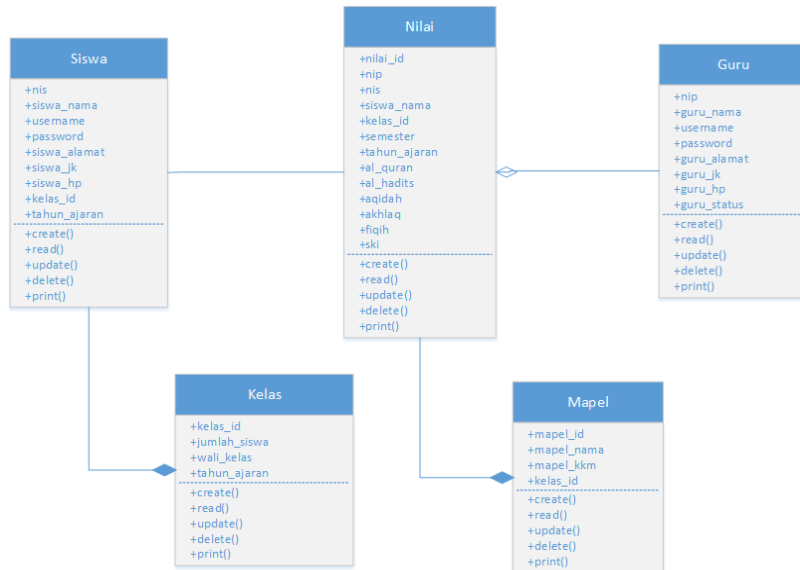
Sumber : Hasil penelitian (2019) Gambar 8 Class Diagram Admin Sistem Pengelohan Nilai Siswa
