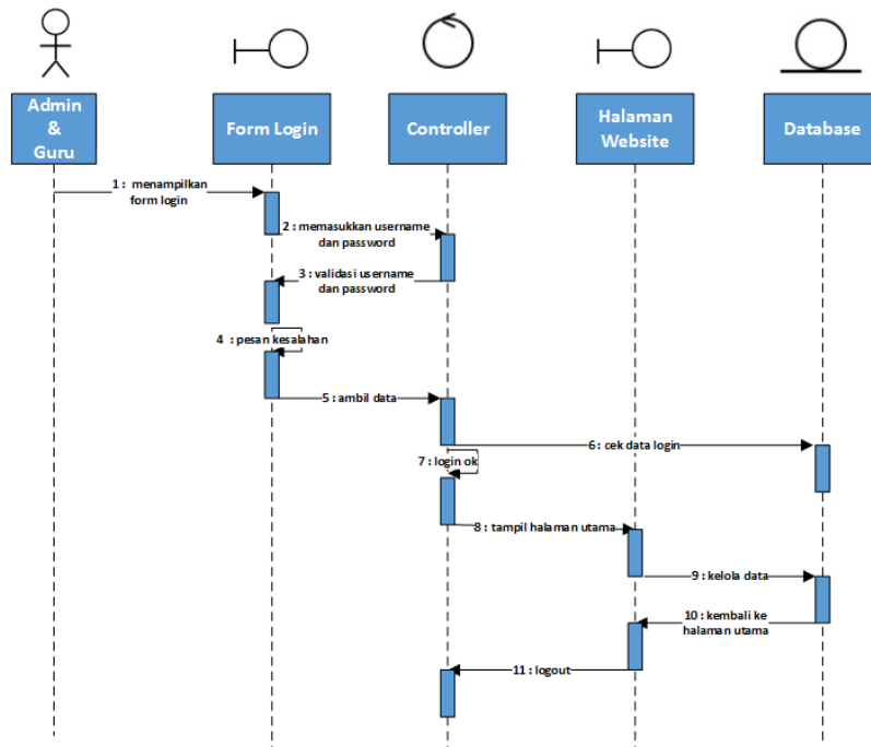
Sumber : Hasil penelitian (2019) Gambar 9 Sequence Diagram Admin dan Guru Sistem Pengelohan Nilai Siswa
