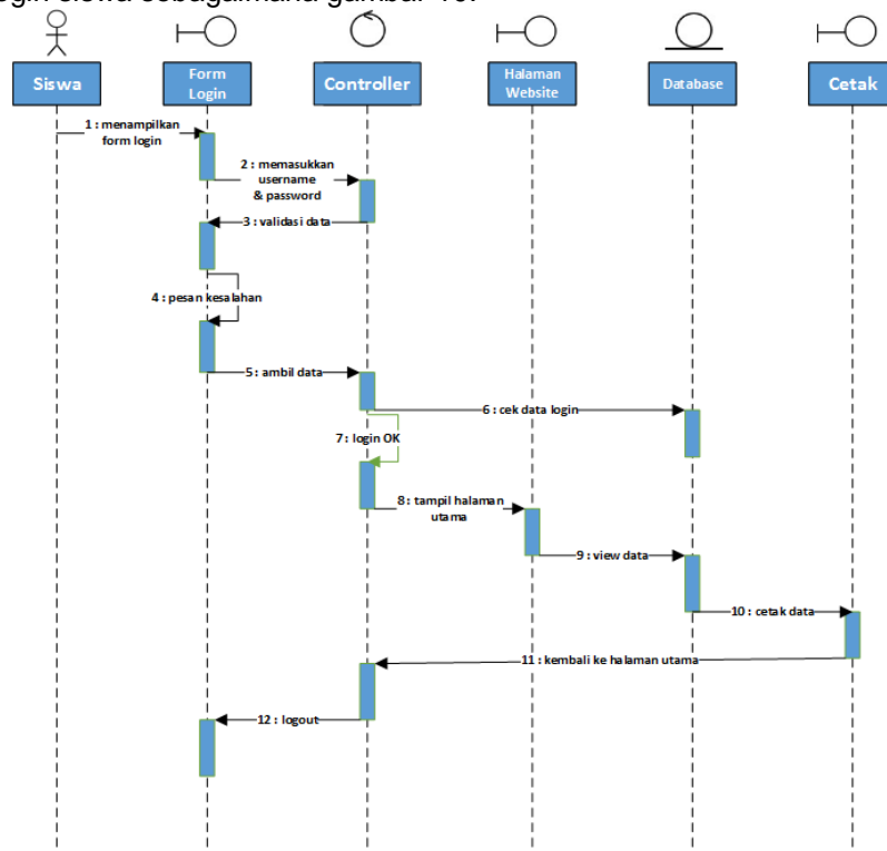
Sumber : Hasil penelitian (2019) Gambar 10 Sequence Diagram Siswa Sistem Pengelohan Nilai Siswa
