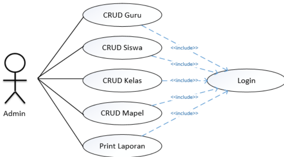
Gambar 3 Usecase Diagram Admin Sistem Pengelohan Nilai Siswa
