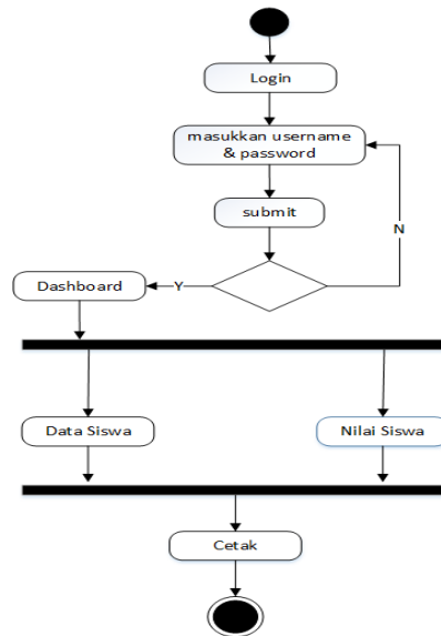
Sumber : Hasil penelitian (2019) Gambar 7 Activity Diagram Siswa Sistem Pengelohan Nilai Siswa
