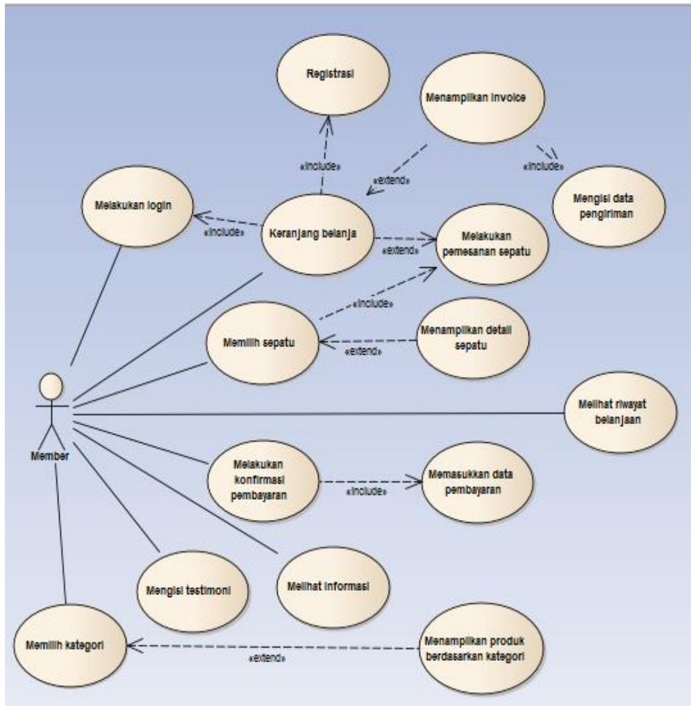
Gambar 2. Use case diagram transaksi penjualan sepatu secara online
