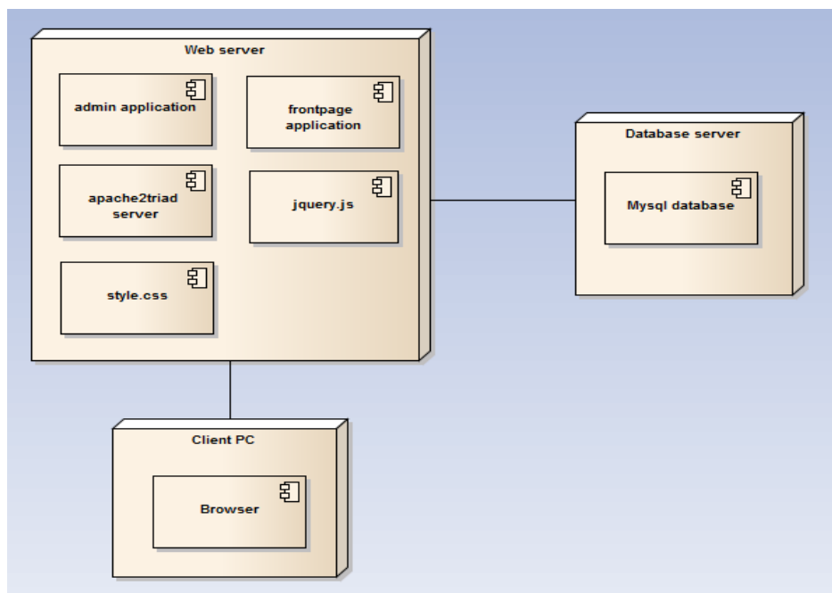
Gambar 7. Deployment diagram pada penjualan sepatu secara online
