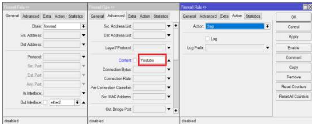
Gambar 6 Pembuatan rule sosial Media
