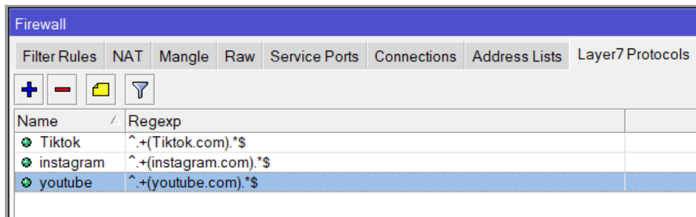
Gambar 5 hasil pembuatan regexp Layer 7 protokol
